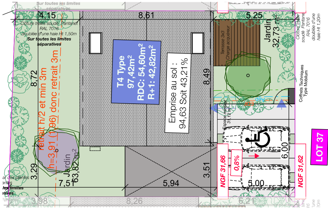
Plan masse
