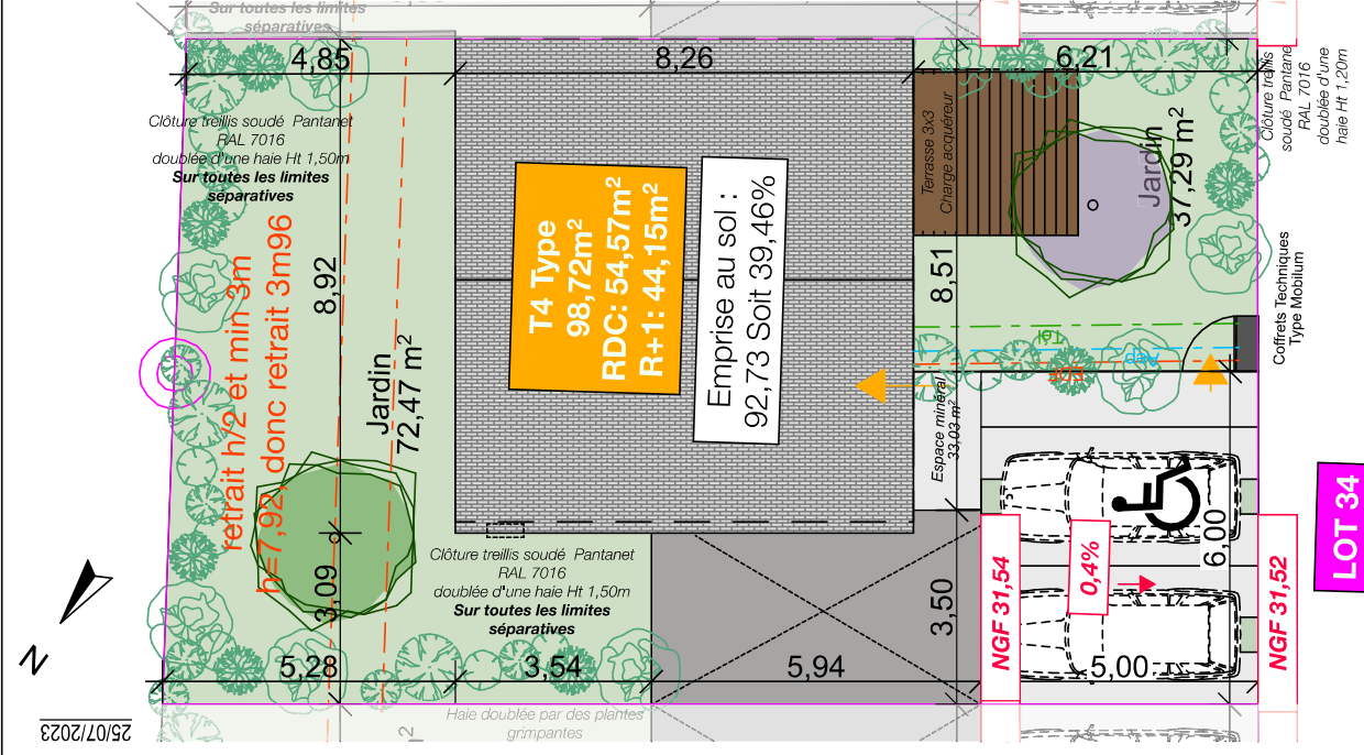
Plan masse
